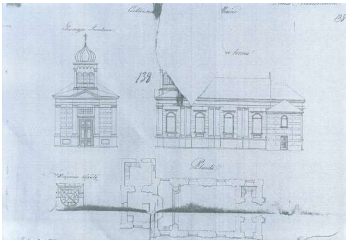
Dokument 1 – Rok 1855, 23 marca/4 kwietnia. Plan budowy cerkwi unickiej w Grabowcu (ze zbiorów Tadeusza Halickiego).
